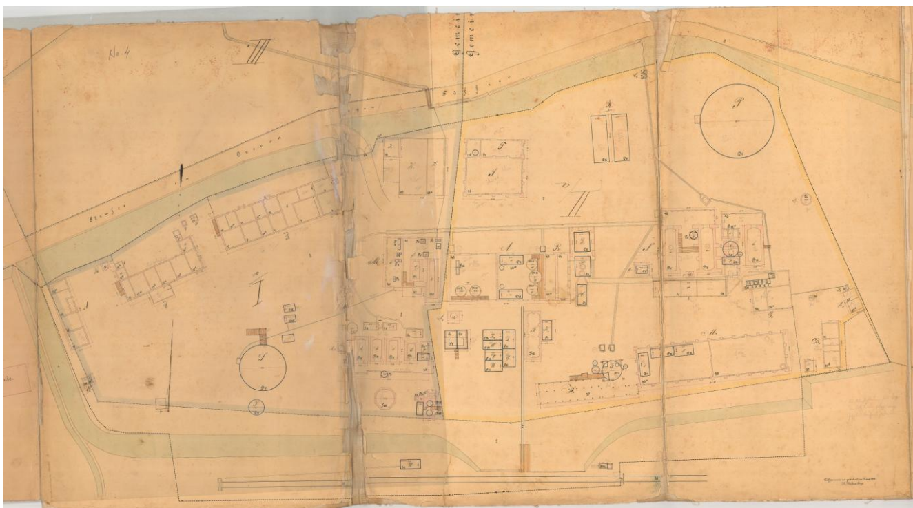
Fig.1. Planul Rafinăriei
