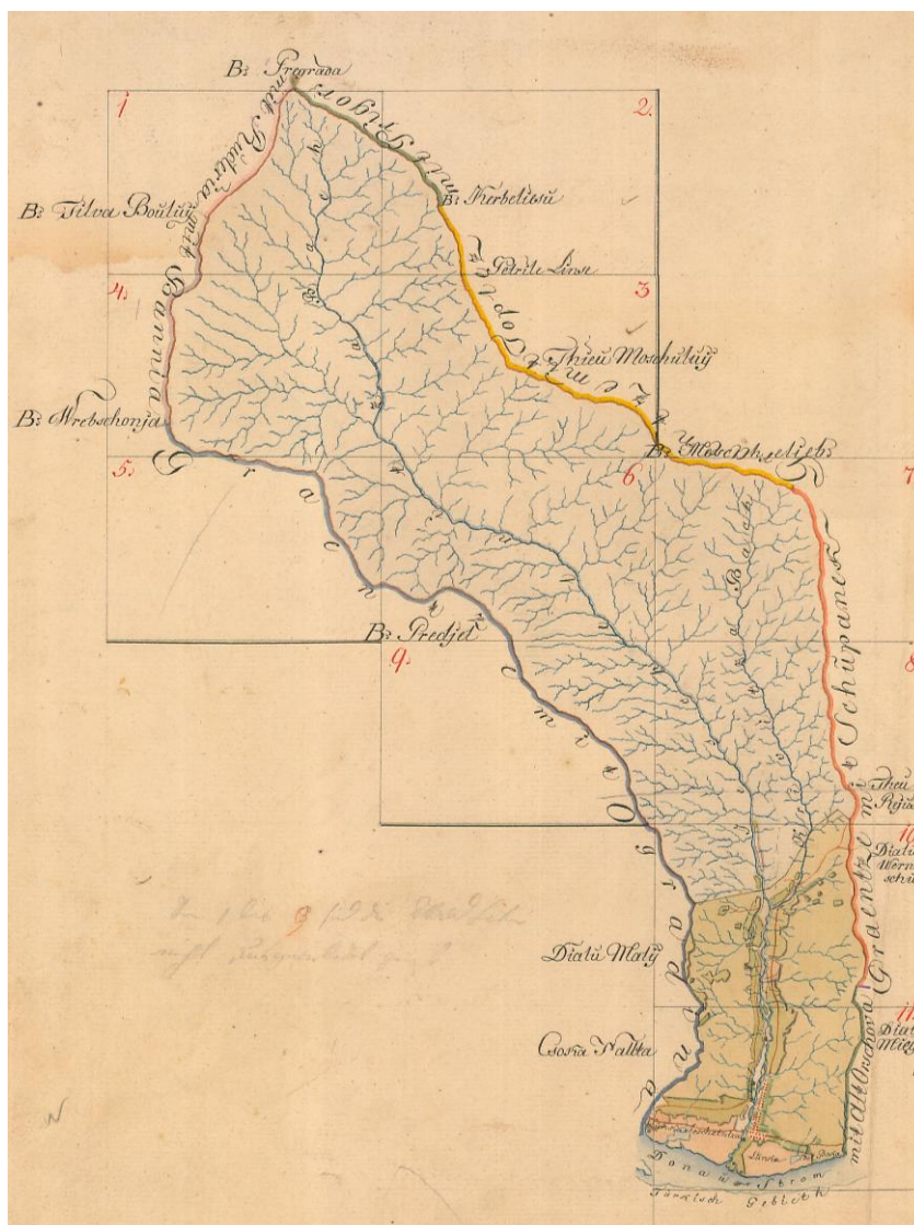
Fig.1. Bazinul hidrografic al leșelniței
